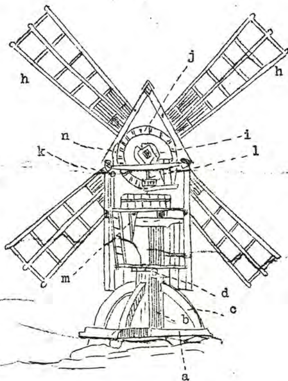
Fig. 10. Väderkvarn. Sektion.
